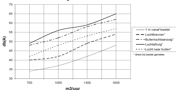
Geluidmeting KB1600CVK
